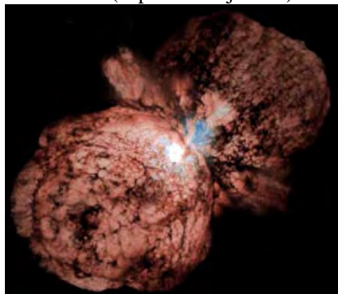
Eta Carinae (supernovan jäänne)
